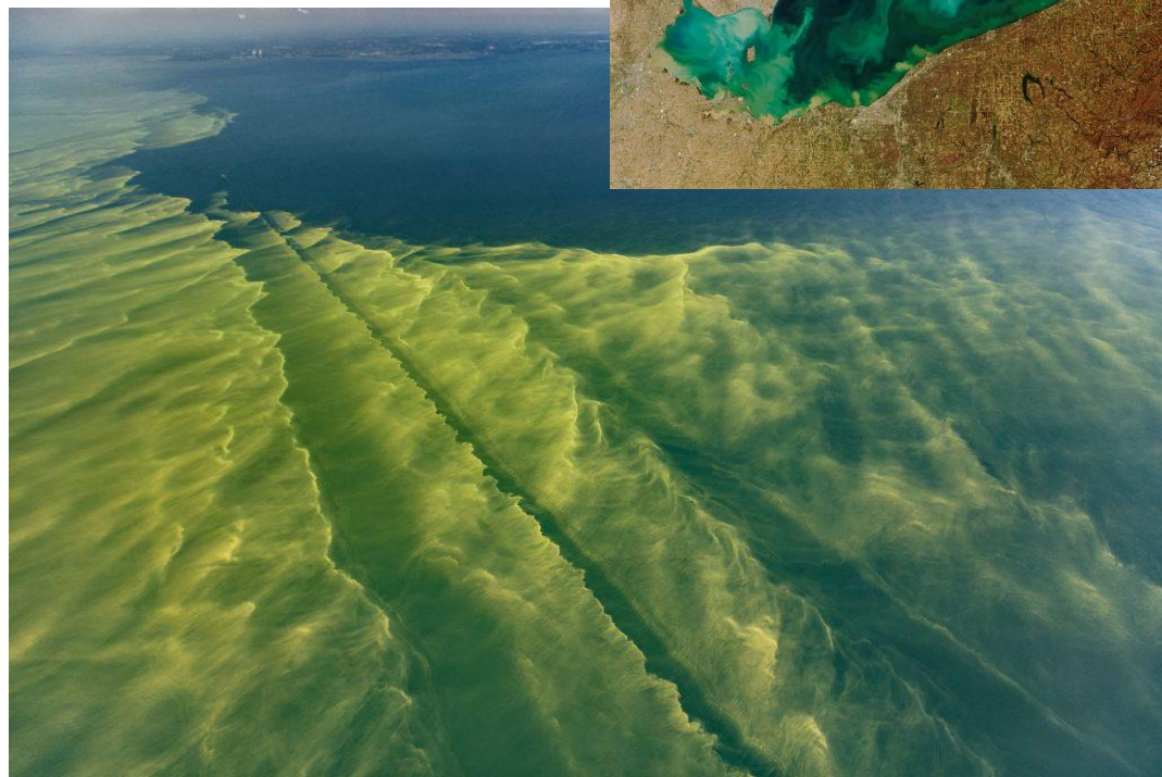
Lake Erie bloom
